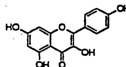
KAEMPFEROL
